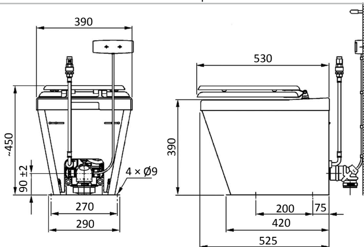
ВУ-ВМ 4, Напольная модель из коррозионностойкой стали
